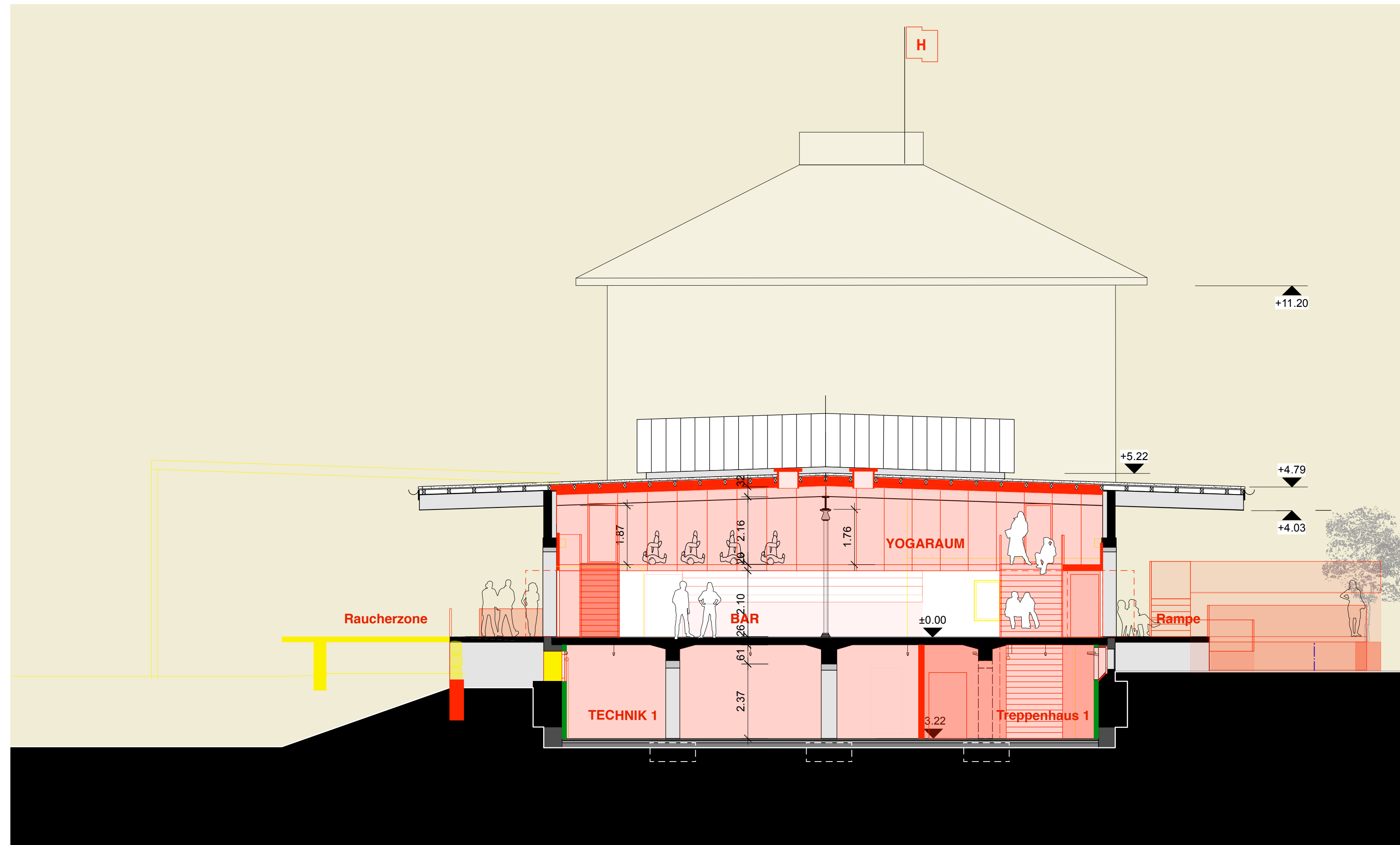
QUERSCHNITT A-A 1 : 100
