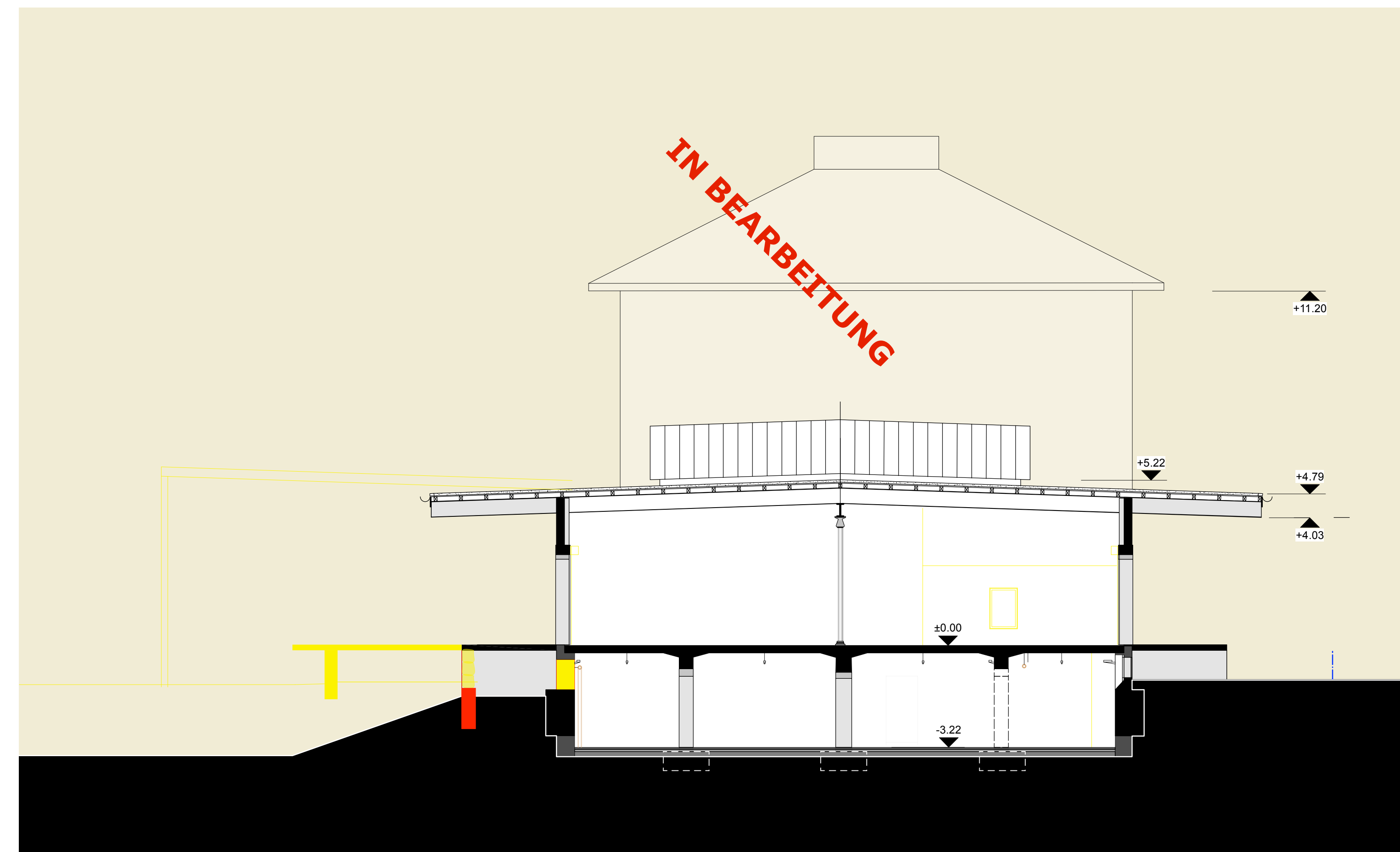
QUERSCHNITT D-D (ANSICHT SÜDWEST) 1 : 100
