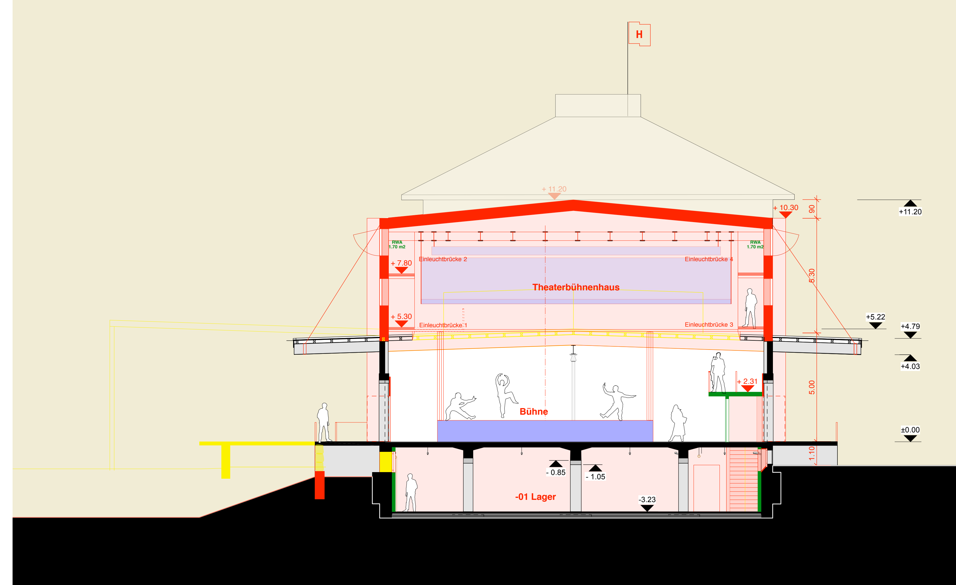
QUERSCHNITT B-B 1 : 100
