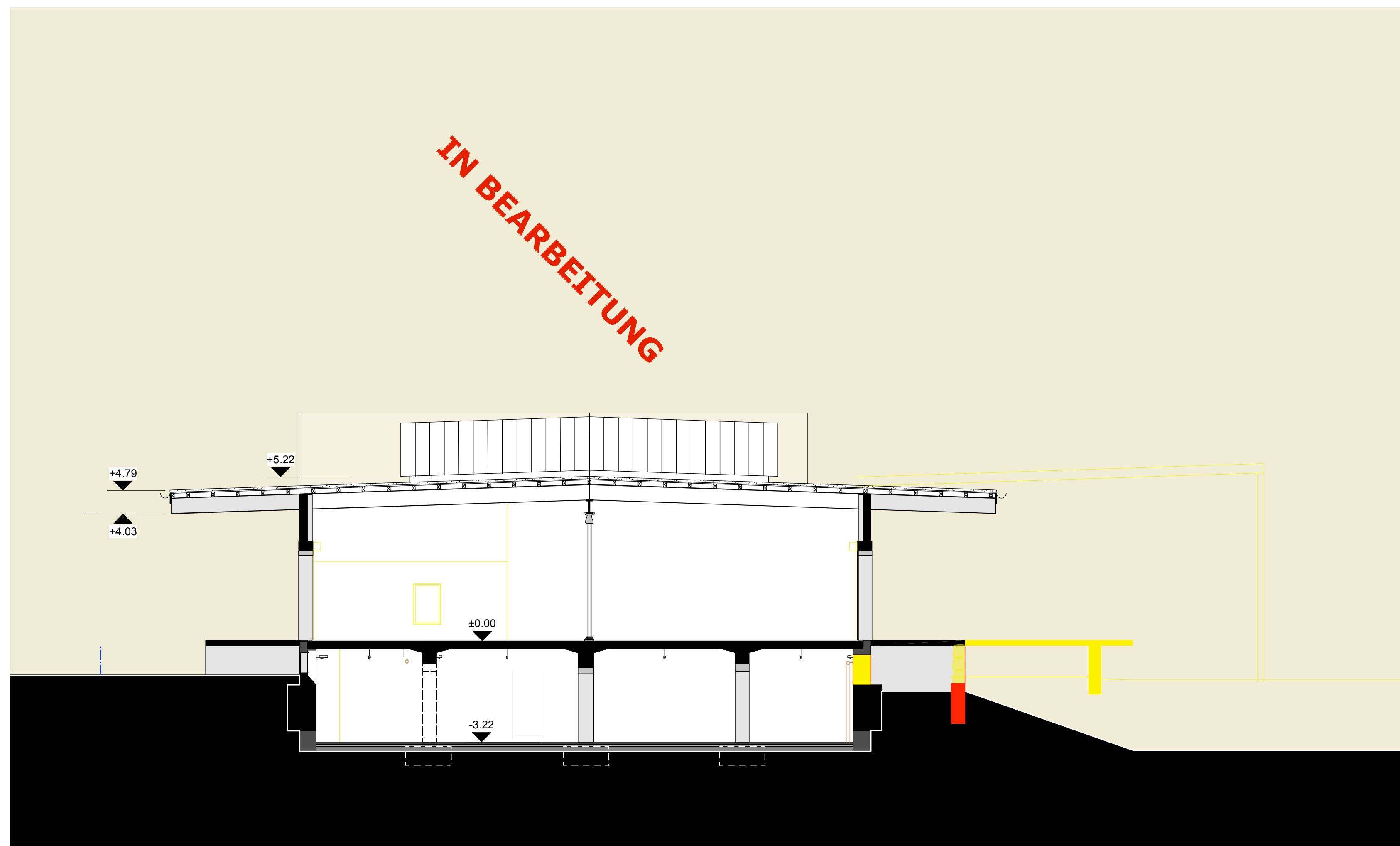
QUERSCHNITT C-C (ANSICHT NORDOST) 1 : 100
