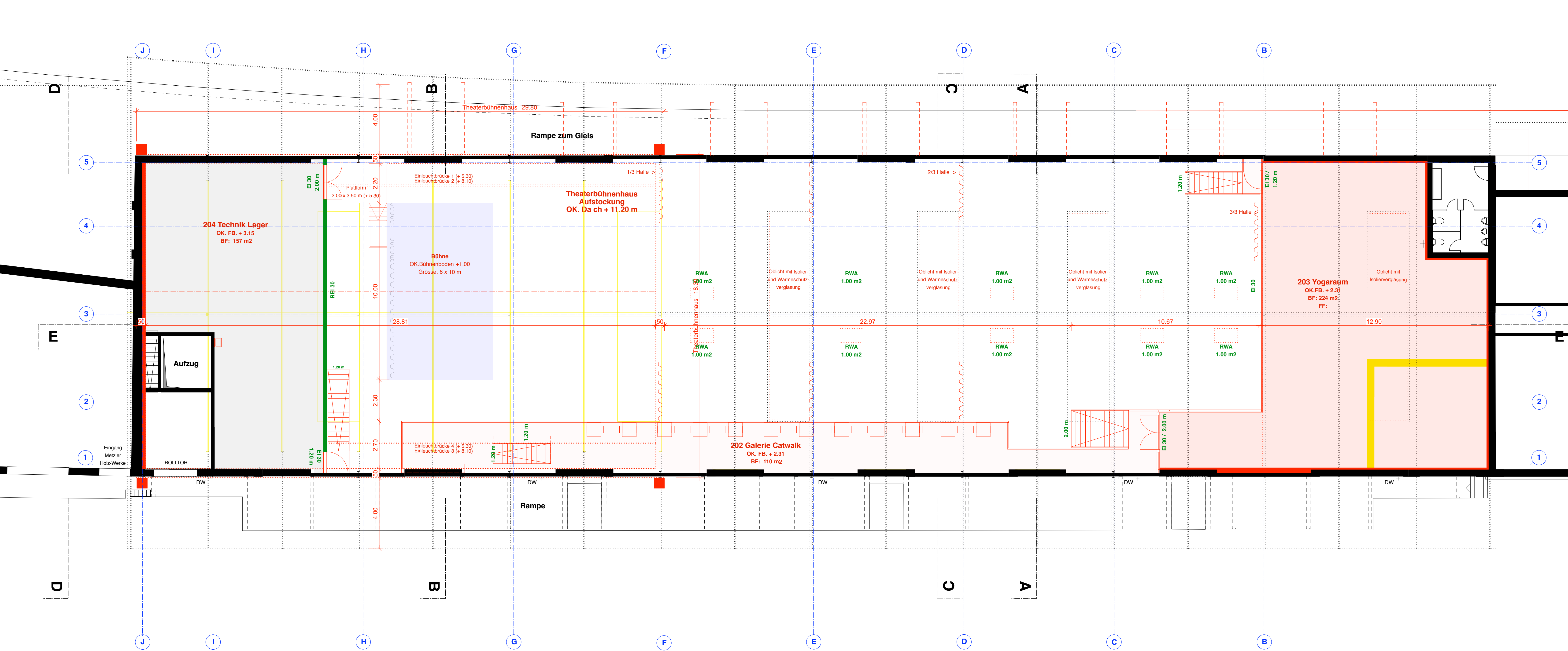
GRUNDRISS Galeriesgeschoss 1 : 100
