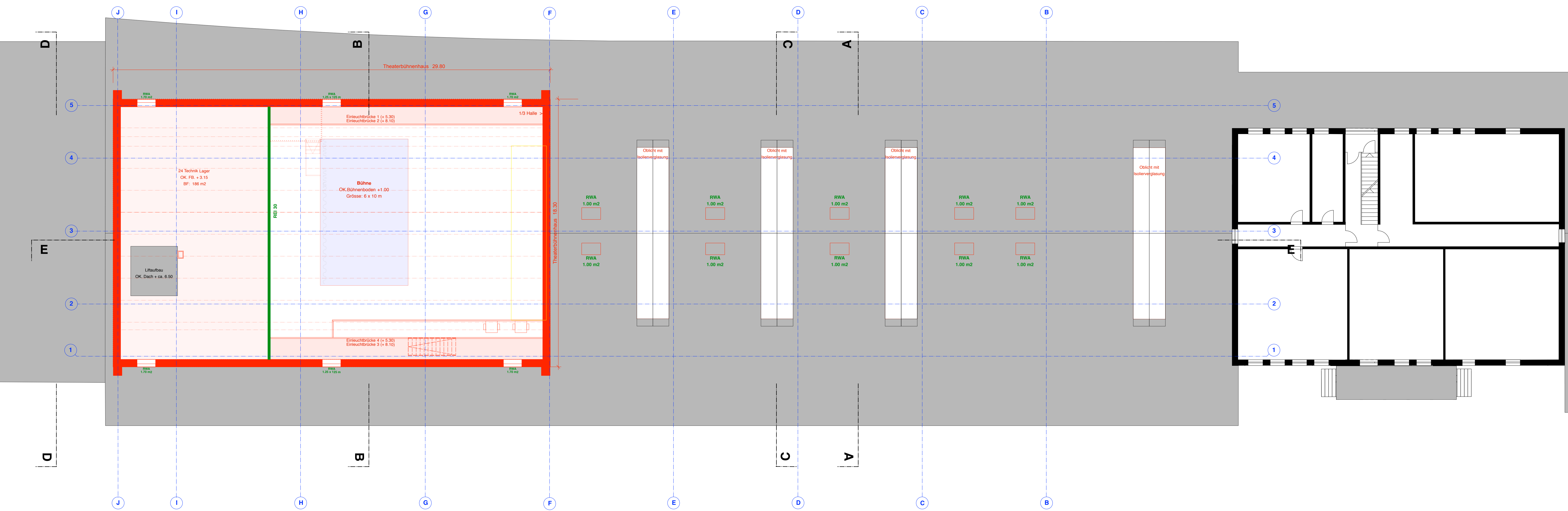
GRUNDRISS Theaterbühnenhaus / Dachaufsicht 1 : 100
