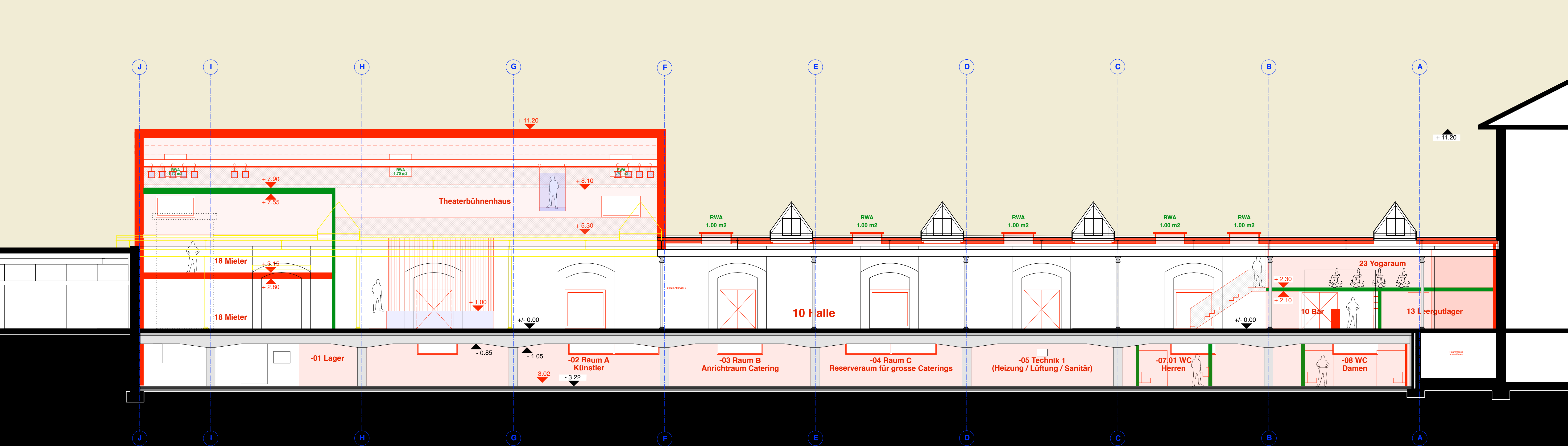
LÄNGSSCHNITT E-E 1 : 100
